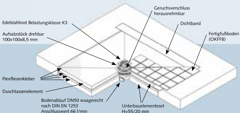
Abb. unten: Schnittdarstellung bei der Version mit waagrechtem Bodenablauf.
